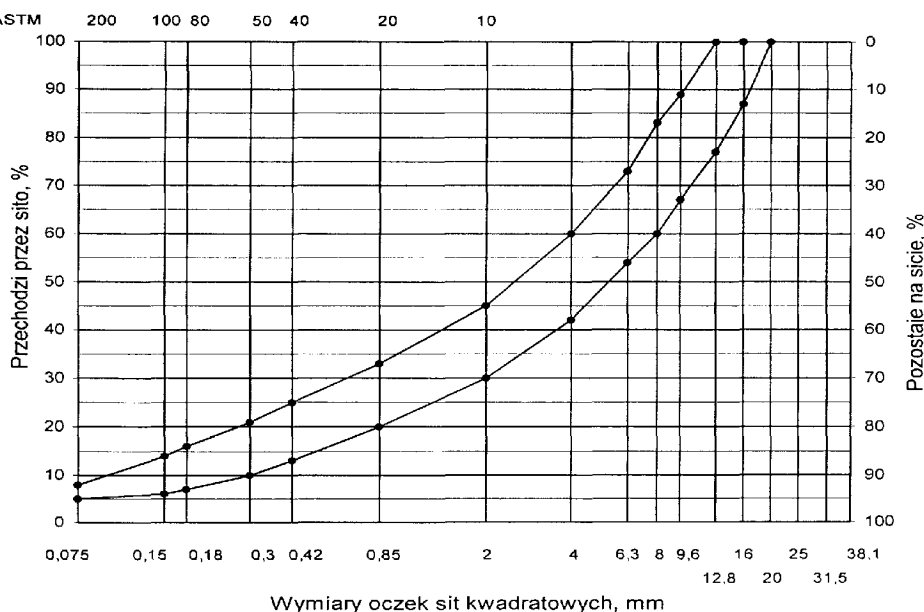
Rys. 6. Krzywe graniczne uziarnienia mieszanki mineralnej BA od 0 do 16 mm do warstwy wyrównawczej nawierzchni drogi o obciążeniu ruchem od KR3 do KR6
