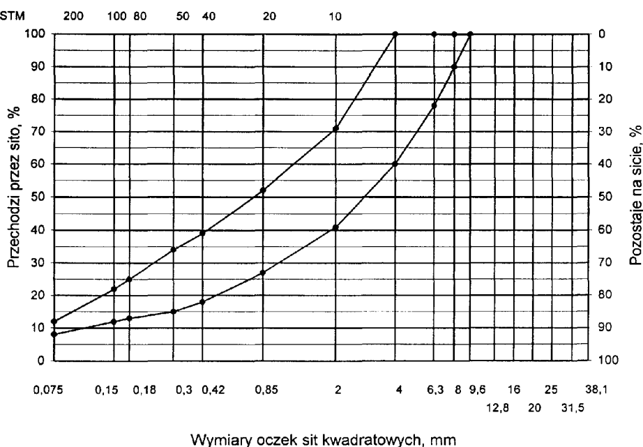
Rys. 1. Krzywe graniczne uziarnienia mieszanki mineralnej BA od 0 do 20 mm do warstwy ścieralnej nawierzchni drogi o obciążeniu ruchem od KR3 do KR6
