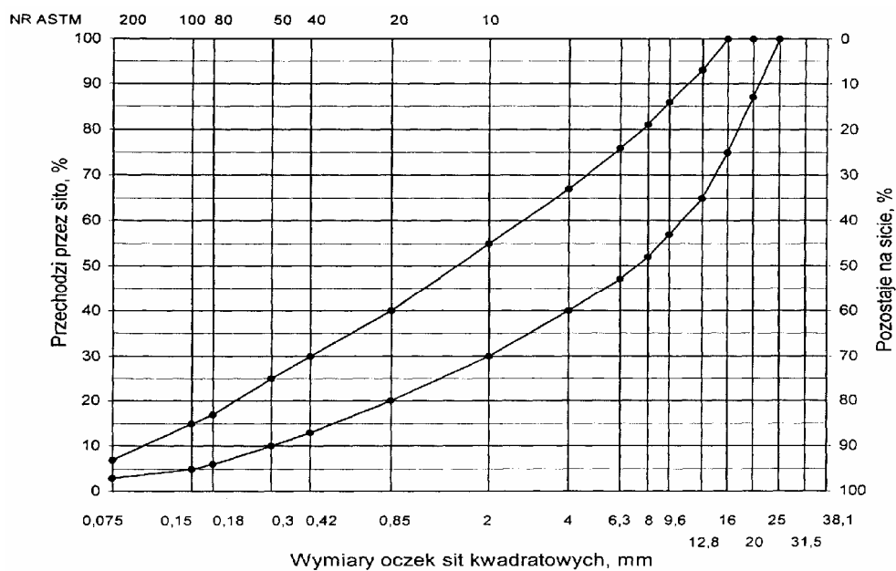
Rys. 8. Krzywe graniczne uziarnienia mieszanki mineralnej BA od 0 do 20 mm.
