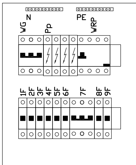
OBUDOWA RWN2x12
